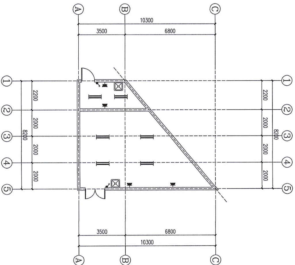
水电平面图
