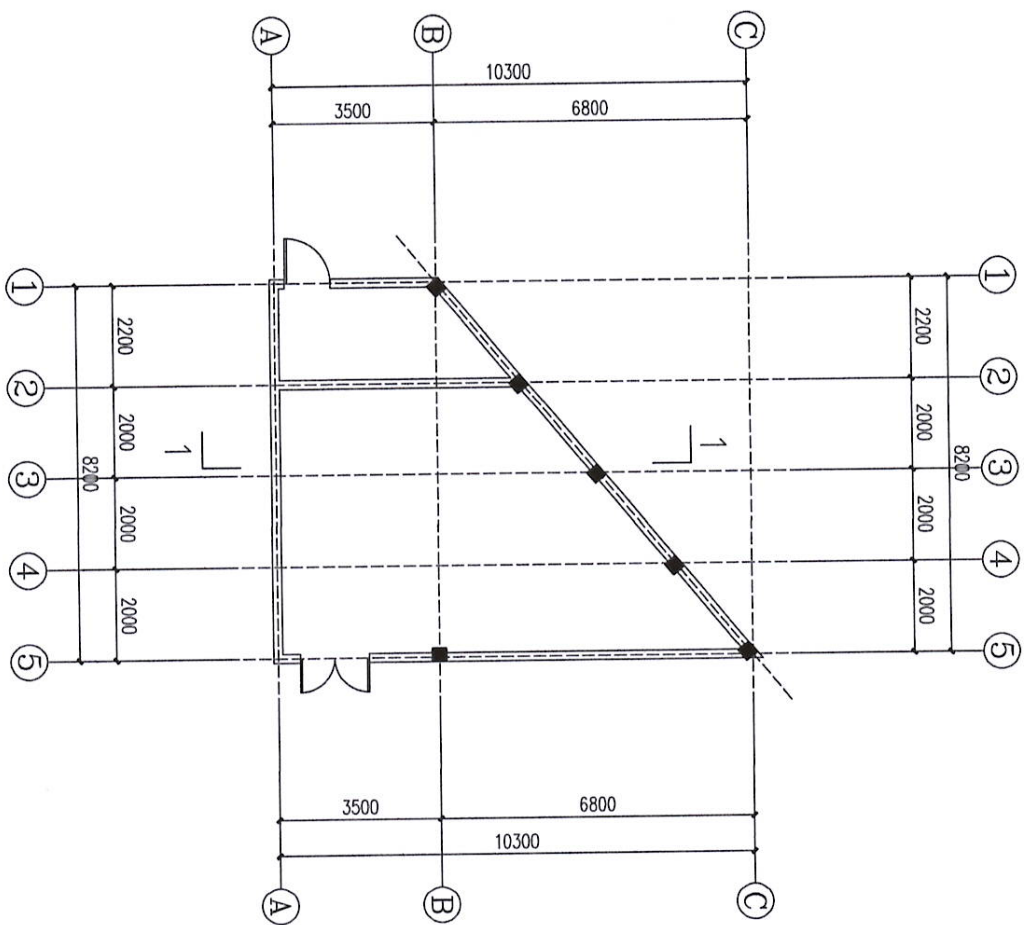
建筑平面图
